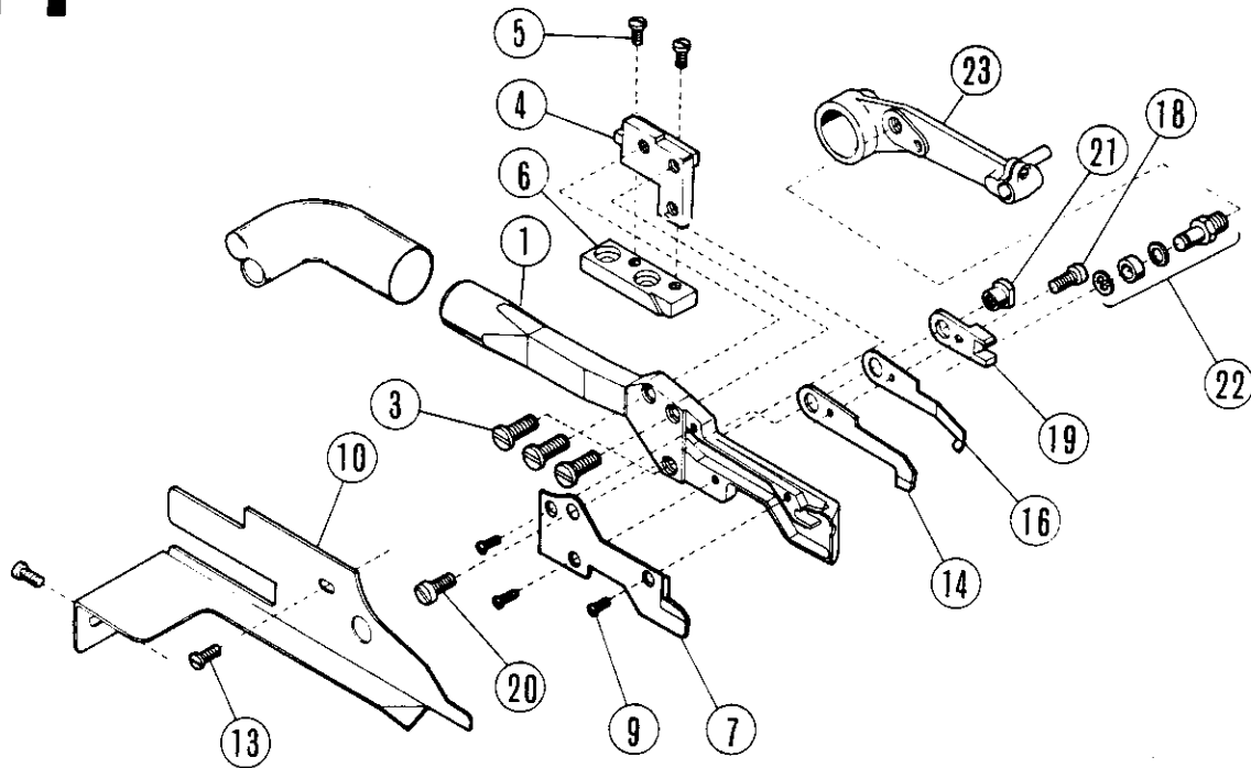
KSR-571 : KSR-572
